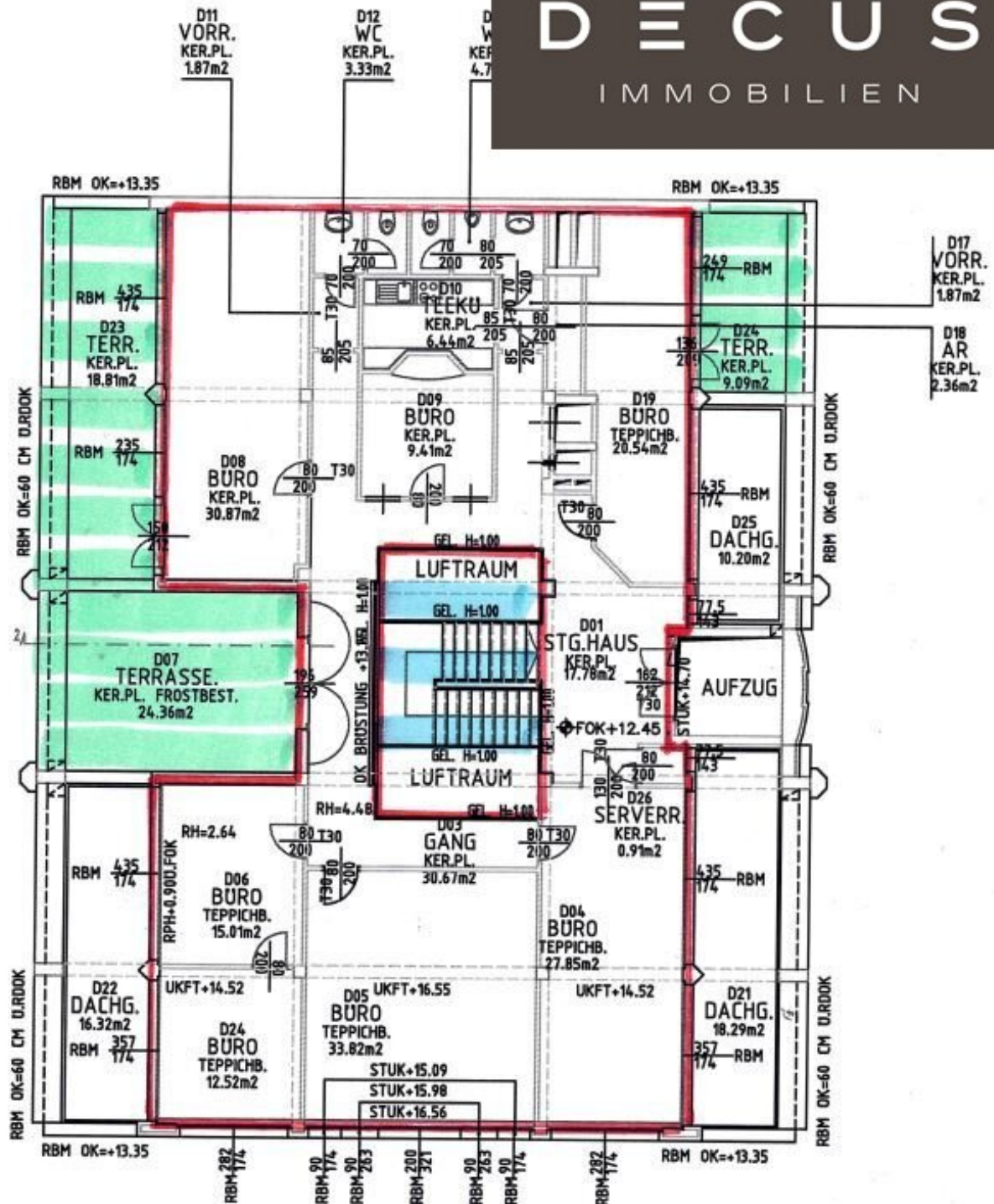
H11 DACHGESCHOSS
