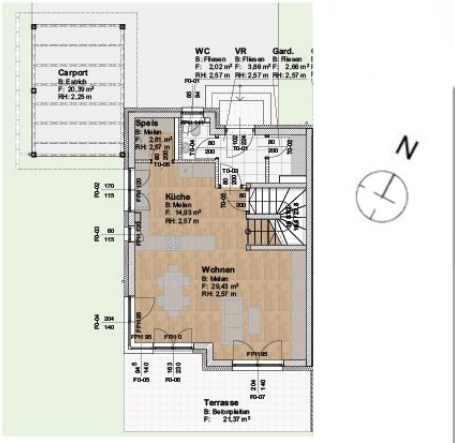
Reihenhausplan | RH 11 Erdgeschoss
