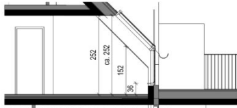
Schnitt 49.A
