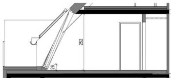
Schnitt 49.B
